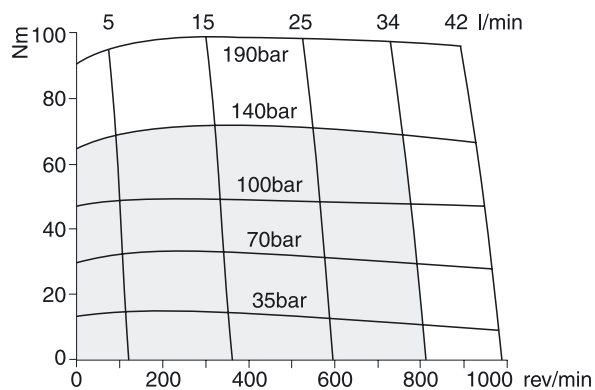
TE/TJ 65
