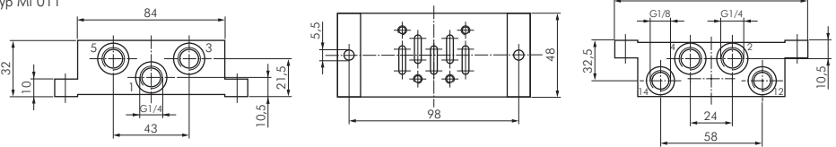
Typ Mi 011
