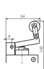
Typ RL 514
