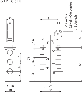
Typ ER 18 510
