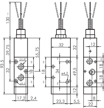
Typ EF 18 510
