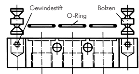
Montagebeispiel
