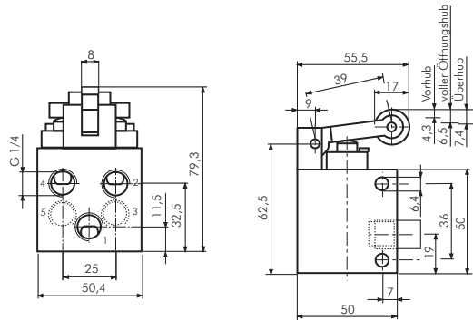
Typ R 514
