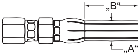
Aussehen der Armaturen 91N nach dem Verpressen
