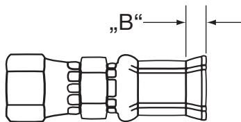
Aussehen der Armaturen 91N nach dem Verpressen
