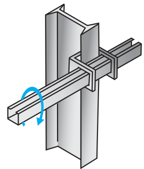
Senkrechte Montage
