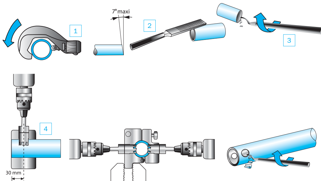
Kronenbohrer für Aluminiumrohr Ref. 6698 02 01
