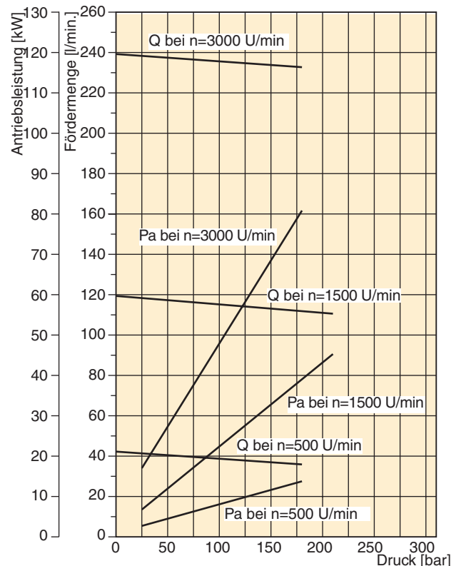
PGP640 - 80,0 cm 3
