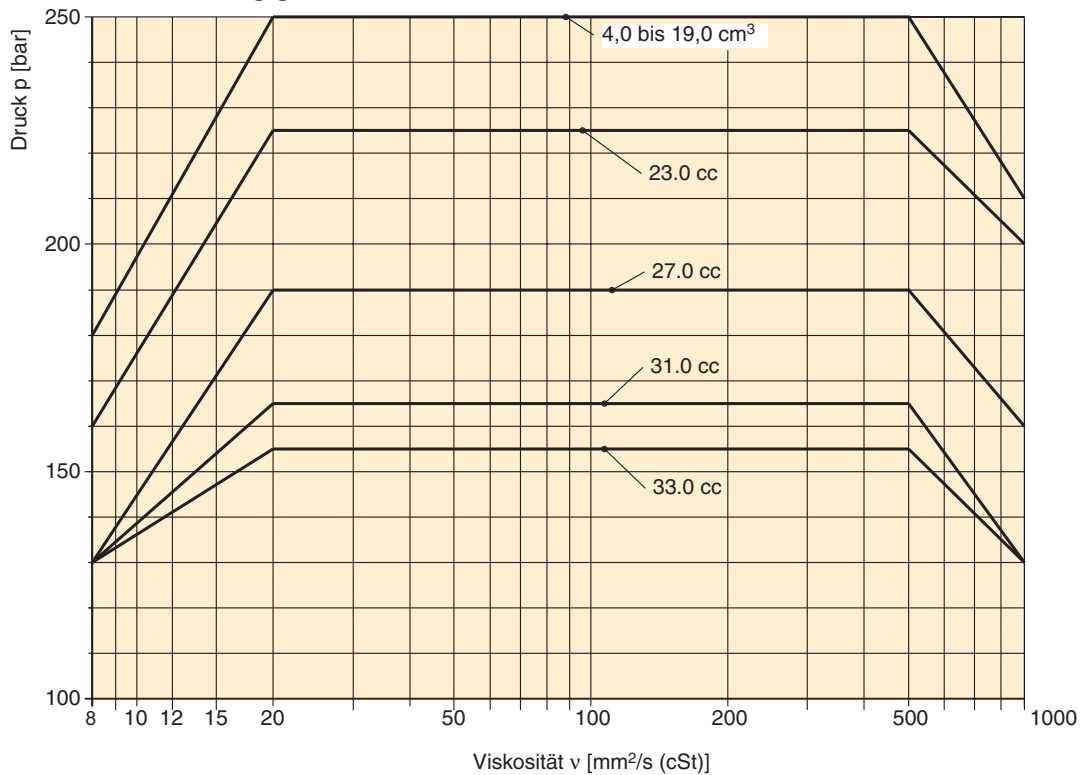
Druck abhängig von Viskosität
