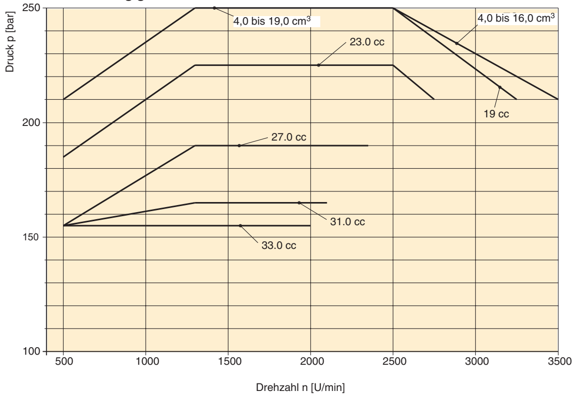
Druck abhängig von Drehzahl
