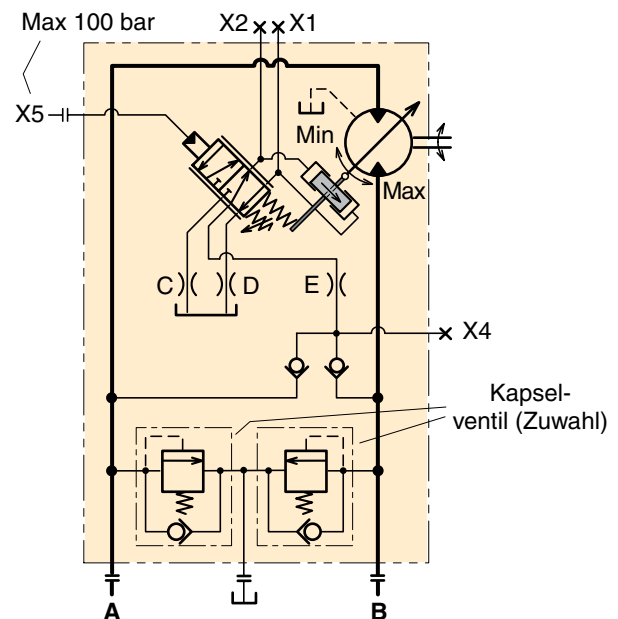
HP-Schaltplan (mit drucklosem Anschl. X5; der Regler bewegt sich zur max. Fördermenge).
