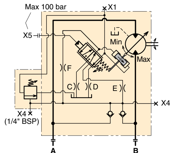
HPC-Schaltplan (mit drucklosem Ansl. X5; der Regler bewegt sich zur max. Fördermenge).
