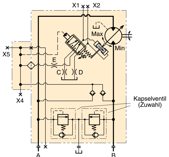
AC-Schaltplan (für Reglerbewegung zur min. Verdr.).
