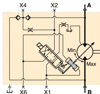
EP H 01 I-Schaltplan (Kolben in ausgeglichener Mittellage).
