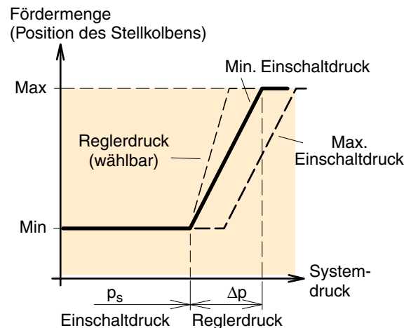
AC-Diagramm (Fördermenge über dem Systemdruck).
