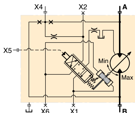
HP S 01 E Schaltplan (Kolben in ausgeglichener Mittellage).
