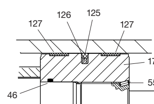
Standard-Kolben
