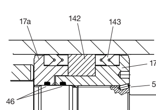
Dachmanschettenkolben
