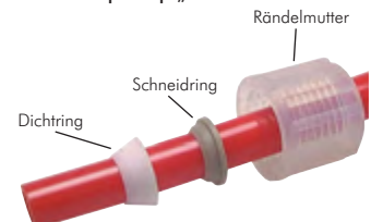
Anschlussprinzip „2“
