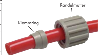
Anschlussprinzip „1“
