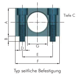
Typ seitliche Befestigung
