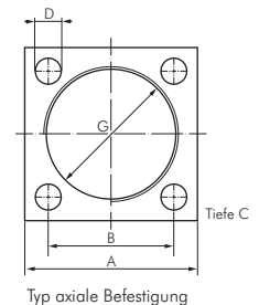
Typ axiale Befestigung
