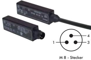
M 8 - Stecker
