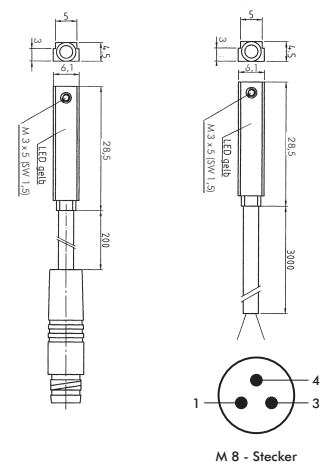
M 8 - Stecker
