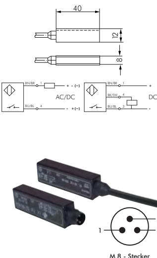
M 8 - Stecker
