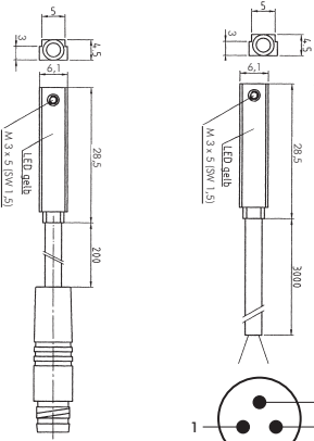
M 8 - Stecker
