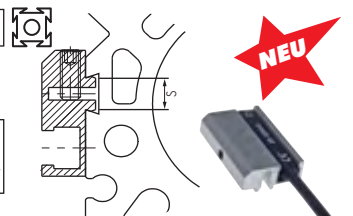
M 8 - Stecker
