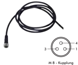
M 8 - Kupplung
